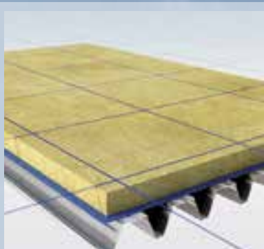
1. Bepaal de plaats van de bevestigingspunten
